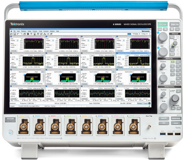
显示在仪器上运行的 SignalVu-PC 多通道 VSA 软件的 MSO68
