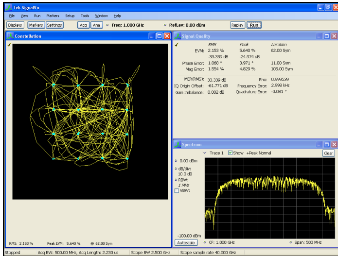
通用数字调制分析功能 (选项 SVM) 用于解调以 312.5 MS/s 运行的 16QAM 回程链路。
