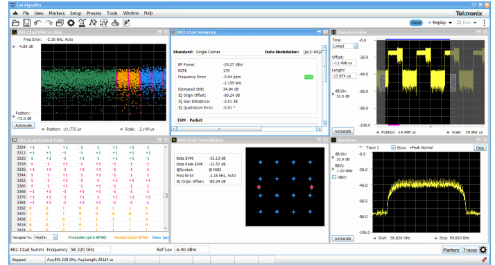
DPO77002SX 及 SV30 提供了业内最佳的 EVM 精度。设置简便，可以执行各种发射机测量，包括突发脉冲的时间概述、频谱、星座图、解码突发脉冲信息和 EVM 测量。
