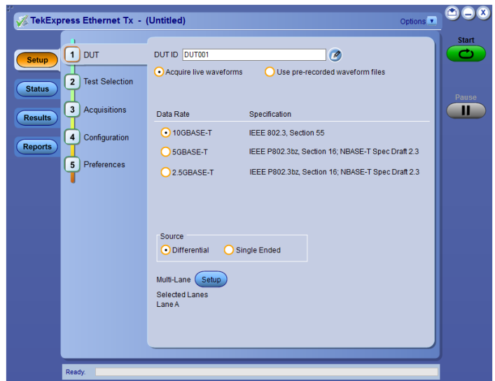
TekExpress 以太网 Tx (选项NBASE-T、XGBT2) - 自动进行10GBASE-T、NBASE-T 和IEEE802.3bz (2.5G/5G) 物理介质连接(PMA) 和物理层(PHY) 电气测试, 为测试以太网设计提供了一种快速且准确的方式。
