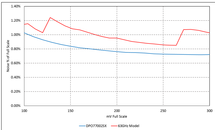
DPO77002SX 与其他厂商的 63 GHz 型号比较：FS 的基本噪声百分比与 mV FS 设置，轨迹居中，60 GHz 带宽，最大采样率设置 (200 GS/s 或 160 GS/s)
