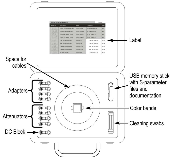
检定 DPO7RFK2-Extended 1.85 mm 的衰减器适配器套件。
