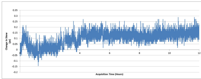
DPO77002SX 系统通道间时延随时间变化。
