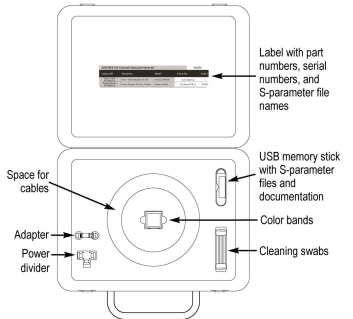
DPO7RFK3-1.85 mm 相差校正套件。
