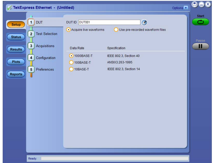
以太网合规性测试解决方案 (选项CMENET3) - 全面的集成式 Tektronix® 以太网工具集, 为10BASE-T、100BASE-TX 和1000BASE-T 以太网提供全面的物理层支持模拟检验、自动化合规性测试软件及设备检定解决方案一应俱全。
