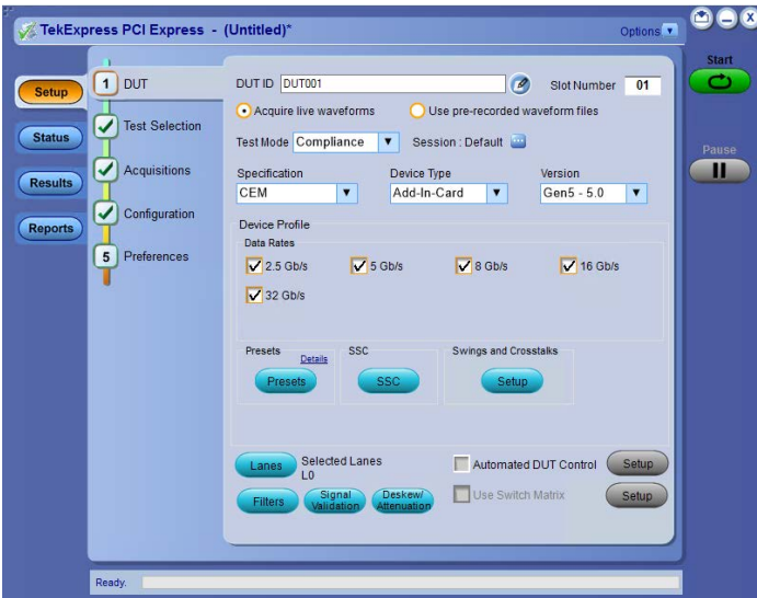
TekExpress® PCI Express Gen 1/2/3/4/5/6 自动化测试软件 (选项PCE3、PCE4、PCE5、PCE6) - 为PCI Express 发射机 (从老式Gen1 到新型Gen6 BASE (截至2022年10月)) 提供最全面的解决方案。包括按照PCI-SIG 规格对PCI Express 装置进行故障排除和验证。应用程序根据测试类型、设备数据速率、发射机均衡、链路宽度和所选探头, 自动选择合适的夹具反嵌和参考通道模拟滤波器及测量选项。TekExpress 包括合规性自动化解决方案, 它将PCI-SIG 的Sigtest 测试软件与泰克基于DPOJET 的PCI Express 抖动和眼图、SDLA 串行数据链路分析可视化工具以及用于Gen6 PAM-4 调制分析的PAMJET 集成在一起。测试结果以综合HTML 格式用于工程测试文档中。
