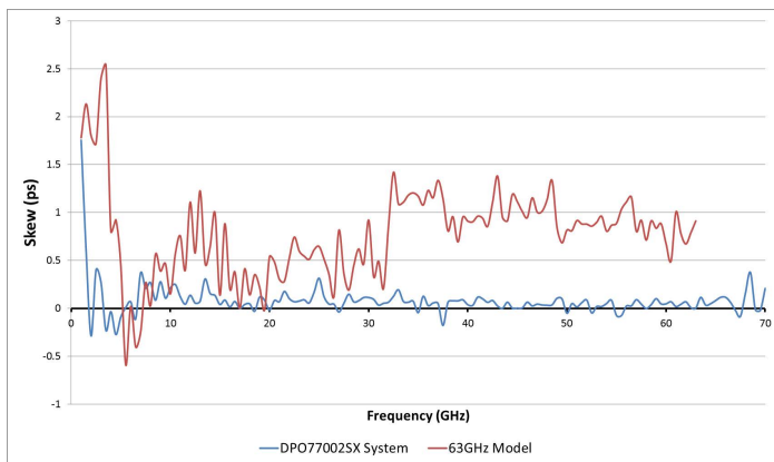
DPO77002SX 系统和另一家厂商 63 GHz 型号的通道时延随频率变化比较。
